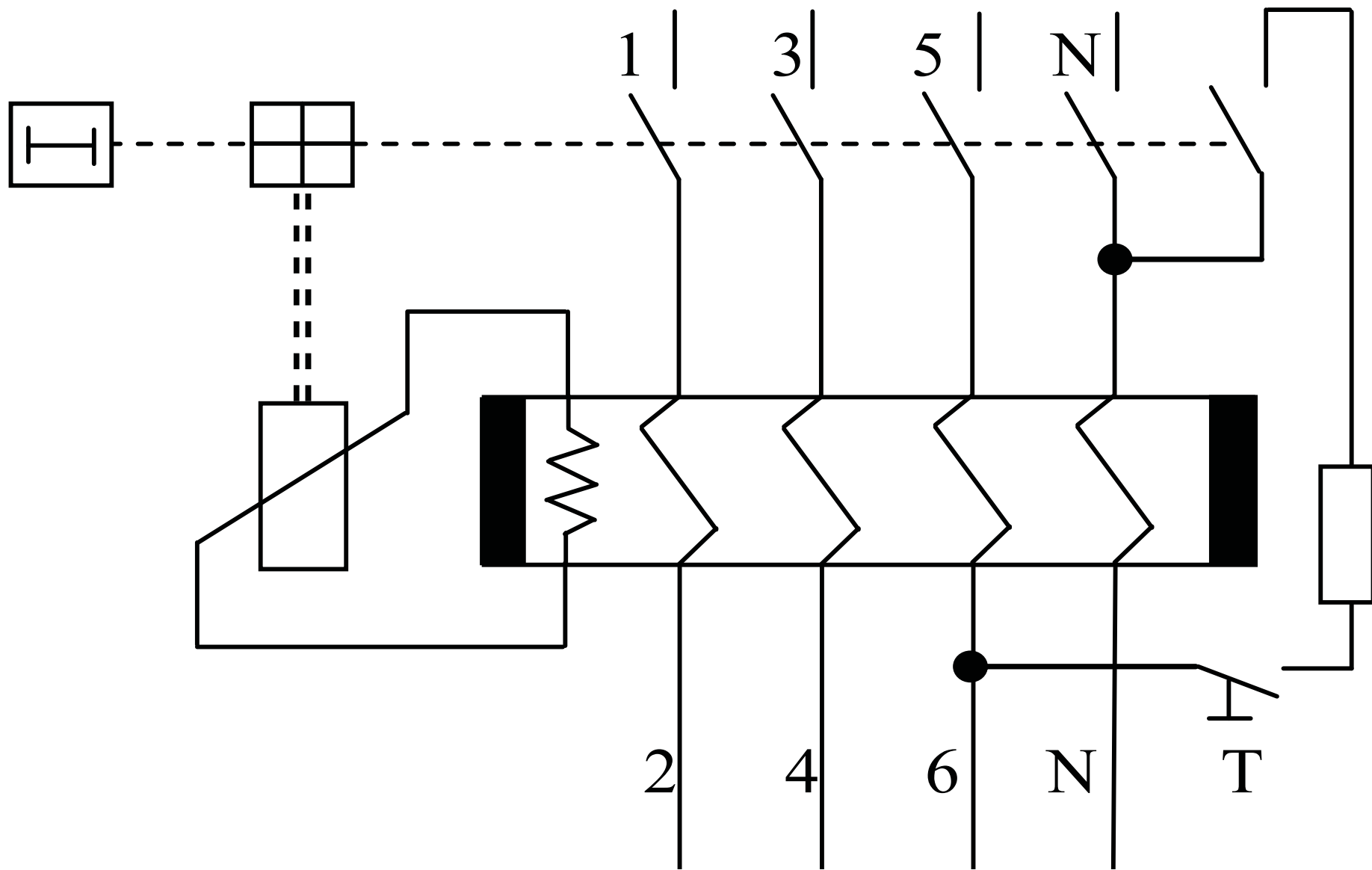
Zapojenie štvorpólového prúdového chrániča
